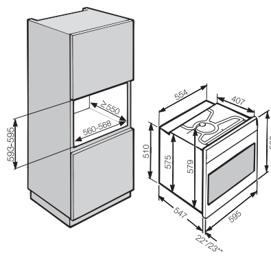
Design de instalação de fornos embutidos
